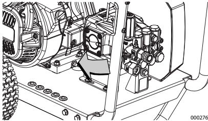
Figura 4-12. Tapón de vaciado de aceite
