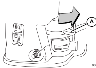
Figure 3-5. Robinet de carburant et étrangleur
