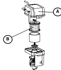
Figura 4-13. Conjunto del filtro de aire
