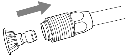
Figura 2-13. Insertar boquilla
