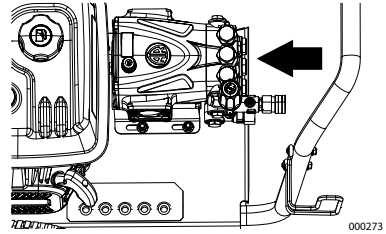
Figura 4-7. Empuje de la bomba hacia el motor
