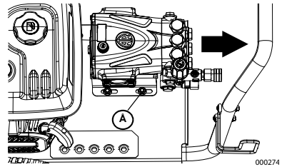
Figura 4-8. Separación de la bomba del motor
